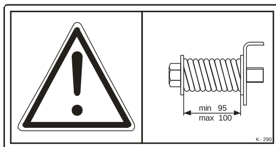
Mechanizm napinania łańcuchów przenośnika podłogowego
