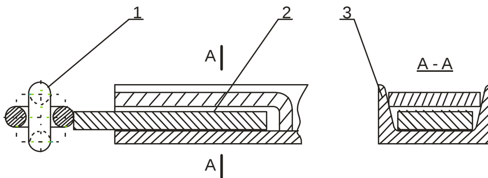
Rys. 2 - Przenośnik podłogowy – fragment łańcucha z listwą.
