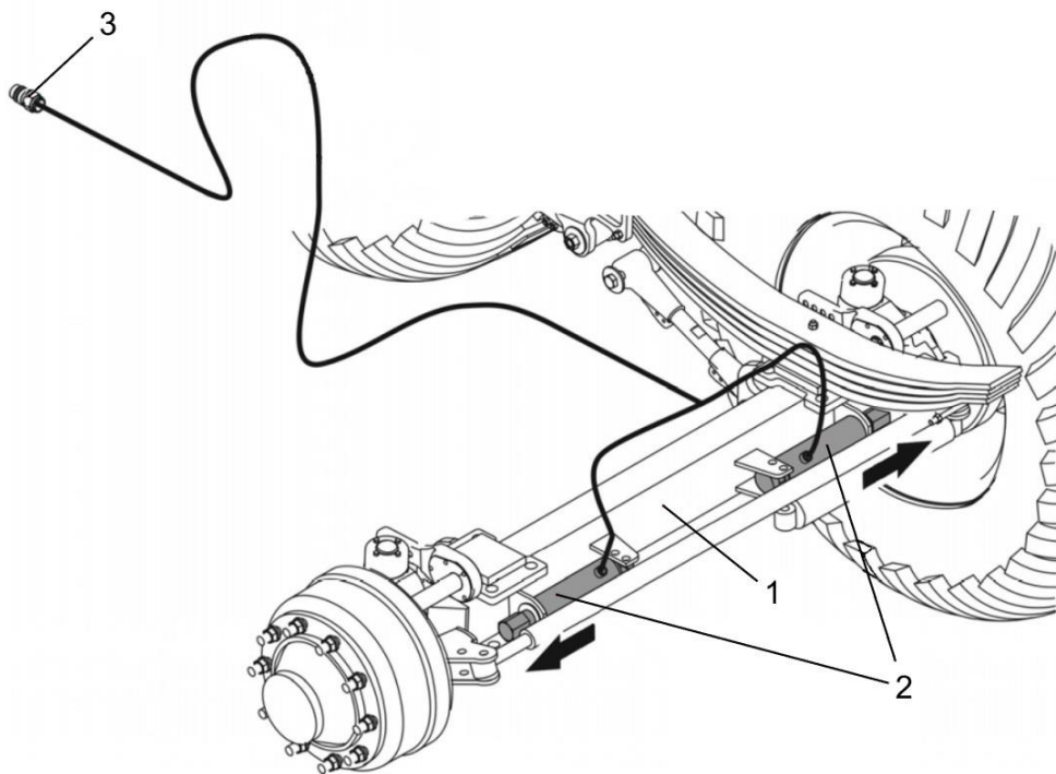
Rys. 11 – Schemat instalacji hydraulicznej blokady kół 1 – skrętna oś jezdnia, 2 – siłowniki hydrauliczne, 3 – szybkozłącze hydrauliczne
