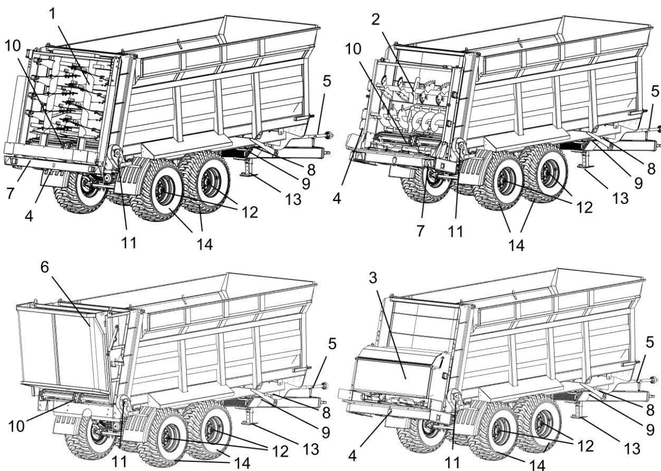
Rys. 24 – Schemat demontażu i kasacji
