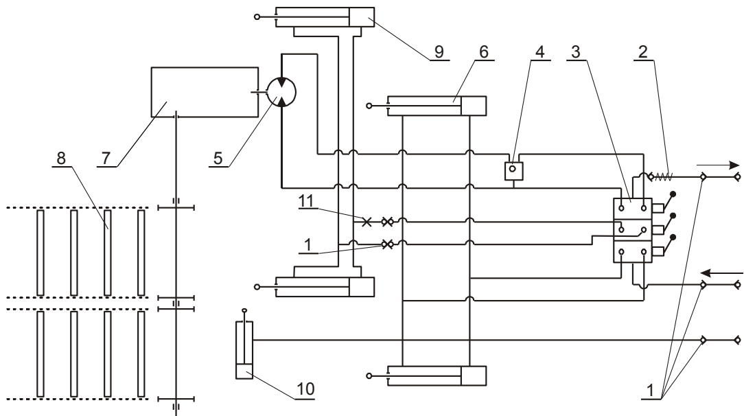
Rys. 10 – Schemat instalacji hydraulicznej (z rozdzielaczem RBS)
