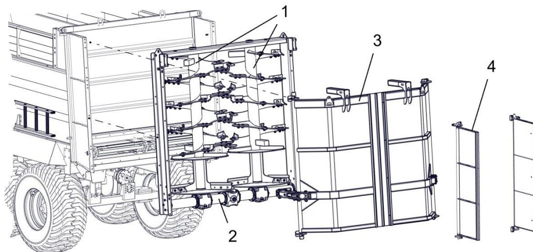
Rys. 17a – Widok poglądowy adaptera pionowego
