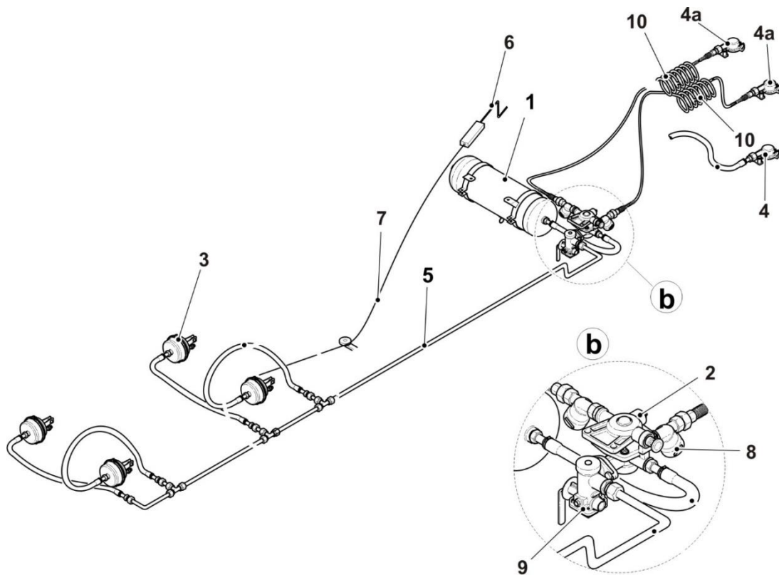
Rys. 3 - Schemat instalacji hamulcowej pneumatycznej jedno- i dwuprzewodowej tandemowej 1 – zbiornik powietrza; 2 – sterownik HZS; 3 – siłownik pneumatyczny; 4 – złącze B2 (do połączenia z instalacją pneumatyczną ciągnika); 4a – złącza instalacji dwuprzewodowej; 5 – przewód powietrzny; 6 – korba hamulca ręcznego; 7 – linka hamulca ręcznego; 8 – filtr powietrza; 9 – regulator siły hamowania; 10 – przewód spiralny
