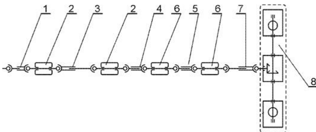
Rys. 17b - Schemat napędu adaptera pionowego dwuwalcowego
