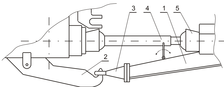
Rys. 15b – Połączenie rozrzutnika z ciągnikiem na zaczep dolny do przyczep jednoosiowych ( hitch )
