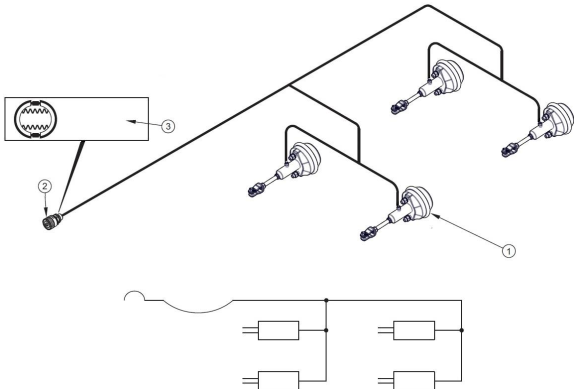
Rys. 5 – Schemat instalacji hamulcowej hydraulicznej tandemowej
