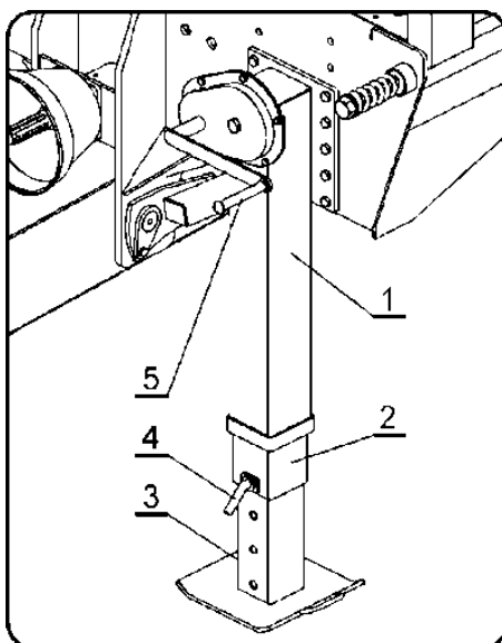
Rys. 14 - Podpora dyszla (dwubiegowa)
