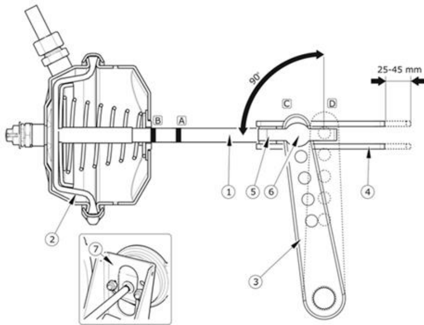
Rys. 6 – Regulacja hamulca
