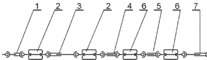
Rys. 1 - Schemat układu przeniesienia napędu
