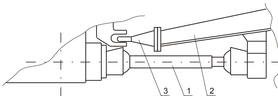
Rys. 15a – Połączenie rozrzutnika z ciągnikiem na zaczep górny
