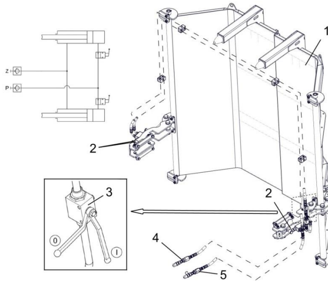
Rys. 21 – Budowa deflektora hydraulicznego oraz schemat instalacji hydraulicznej 1 – klapa tylna, 2 – cylindry hydrauliczne, 3 – zawór odcinający, 4 – przewód zasilający, 5 – przewód powrotny
