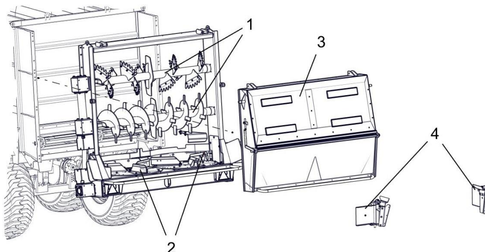
Rys. 18a – Widok poglądowy adaptera poziomo - tarczowego
