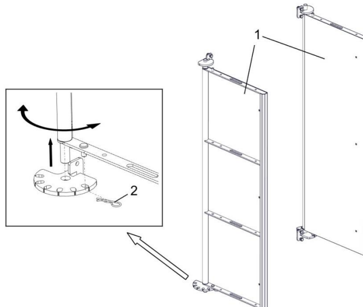
Rys. 22 – Deflektor mechaniczny 1 – Ściany boczne, 2 – zawleczka zabezpieczająca
