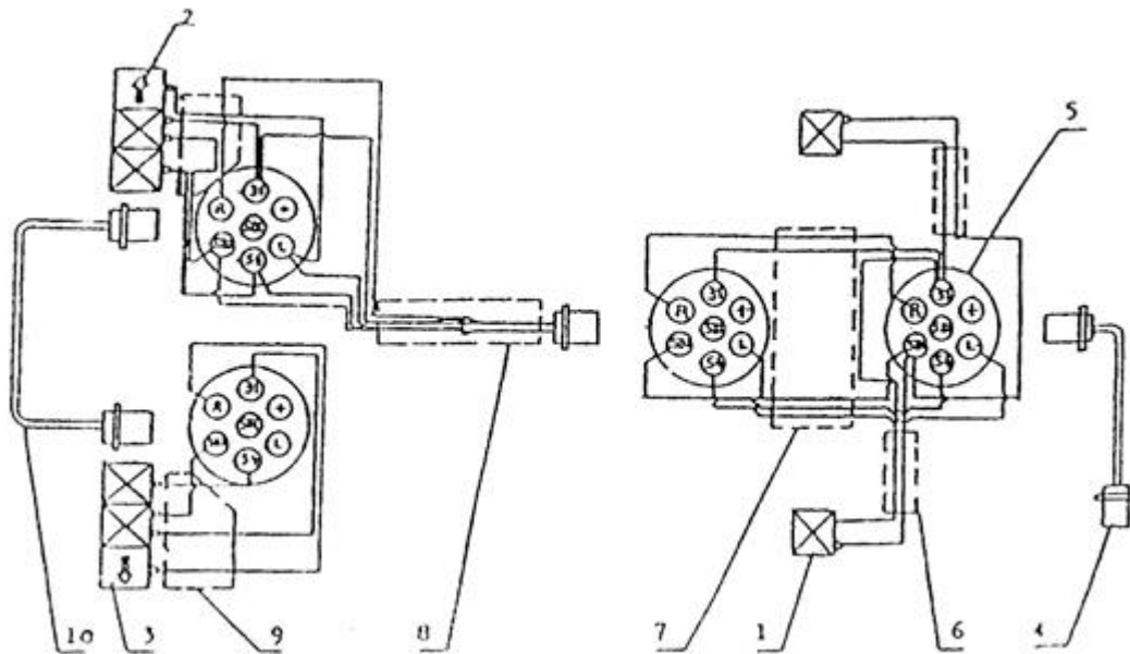
Rys. 13 – Elementy oświetlenia i sygnalizacji
