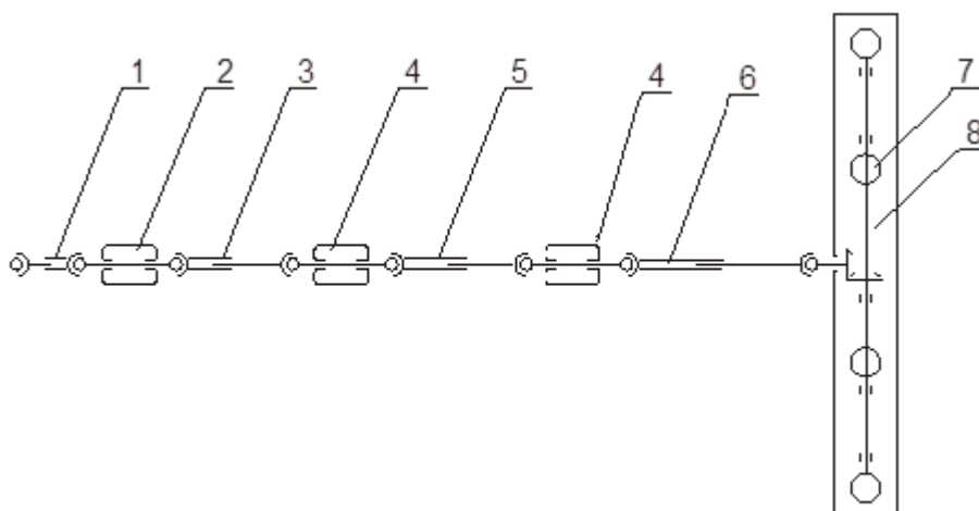
Rys. 16b – Schemat napędu adaptera pionowego czterowalcowego
