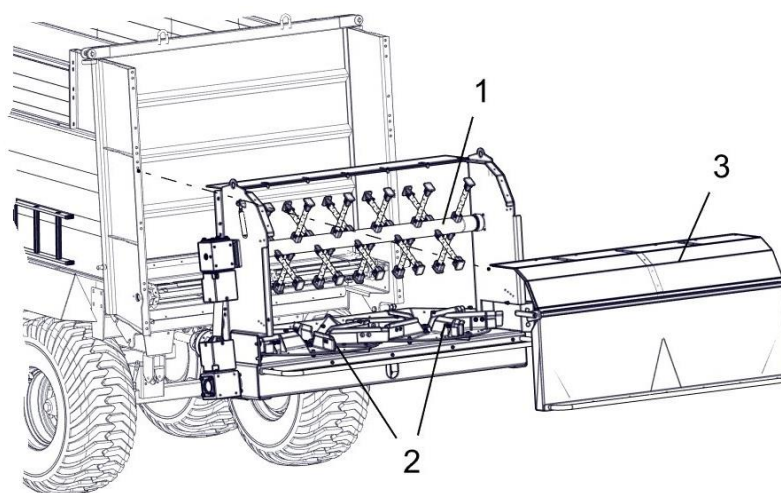
Rys. 19 – Adapter rozdrabniająco – tarczowy
