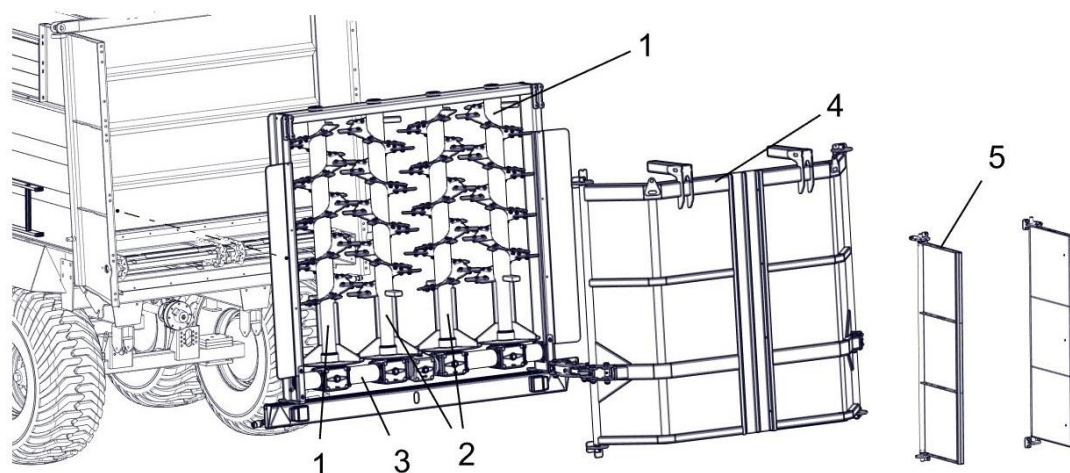
Rys. 16a – Adapter pionowy czterowalcowy
