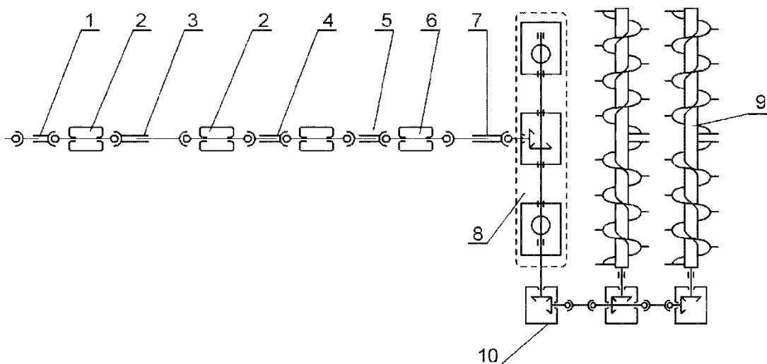
Rys. 18b – Schemat napędu adaptera poziomo - tarczowego
