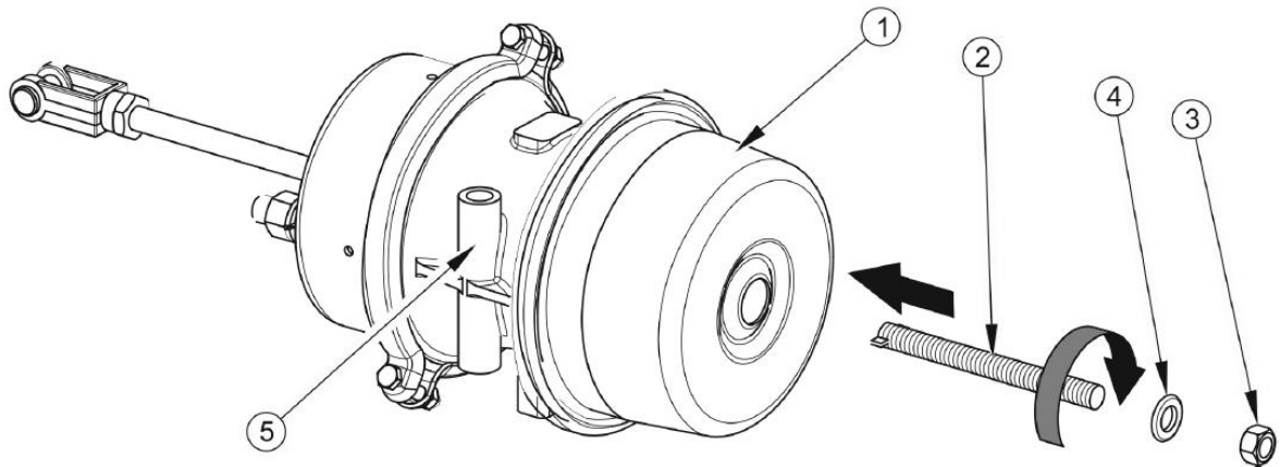
Rys. 7 – Awaryjne zwalnianie siłownika membranowo – sprężynowego.
