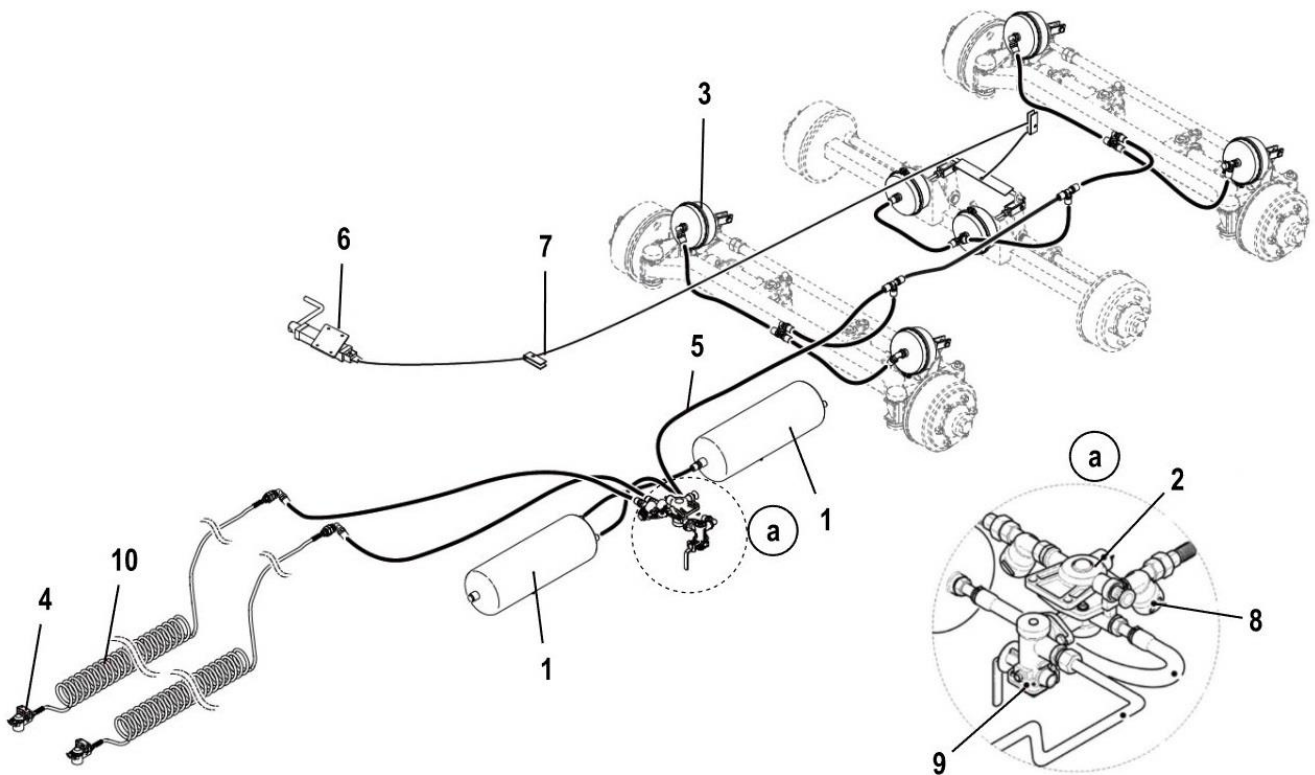
Rys. 4 - Schemat instalacji hamulcowej pneumatycznej dwuprzewodowej tridemowej
