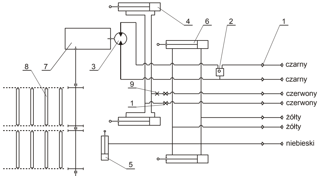
Rys. 9 – Schemat instalacji hydraulicznej (standard)
